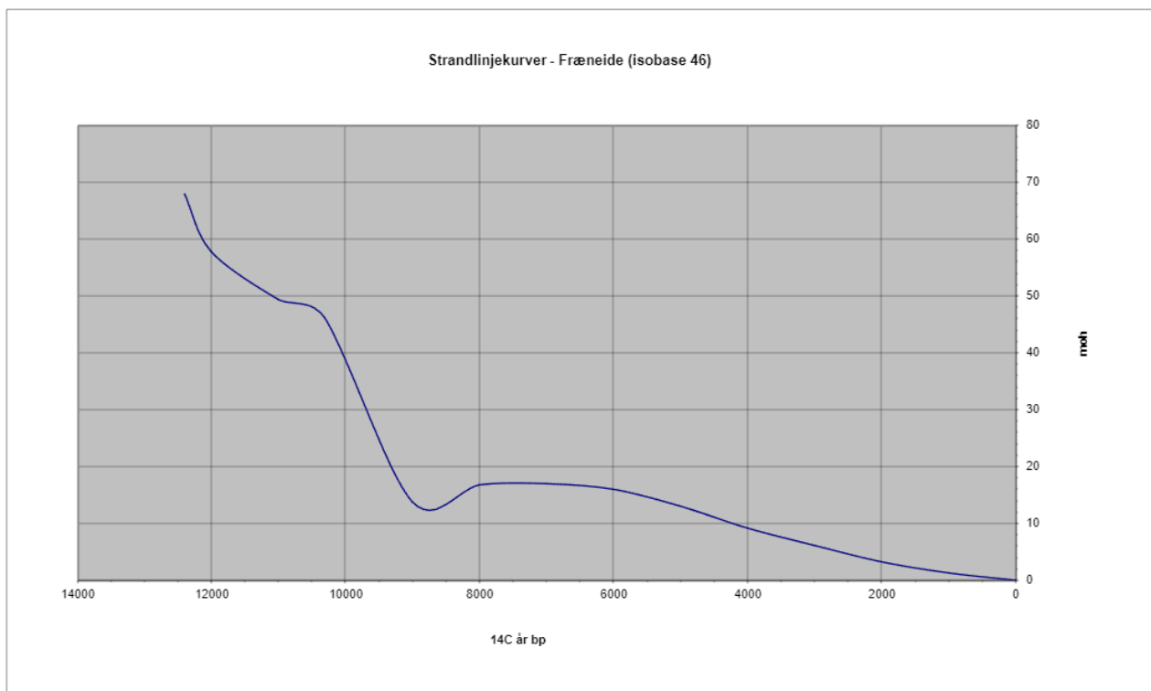
Figur 6. Strandlinjekurve for Fræneide i Hustadvika kommune etter skjema utarbeidet av David N. Simpson, mars 2001 (jf. Svendsen & Mangerud 1987, Bondevik, Svendsen og Mangerud 1998).
