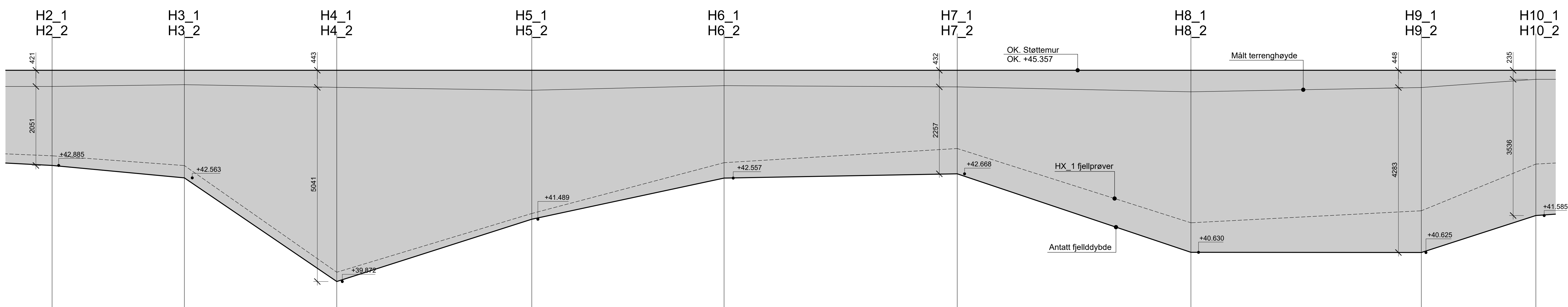
Oppriss av prosjertert støttemur. Antatt dybde er beregnet ut fra målte fjelldybder.
