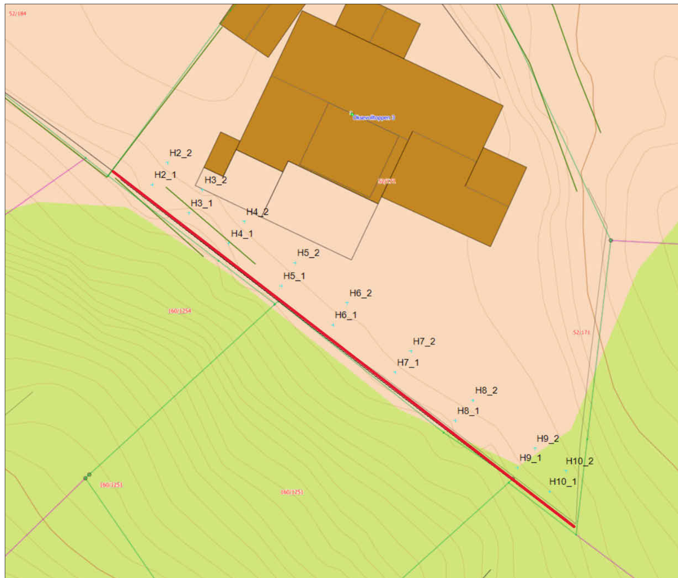
Plan av målte fjelldybder og plassering av ny mur (rød linje).
