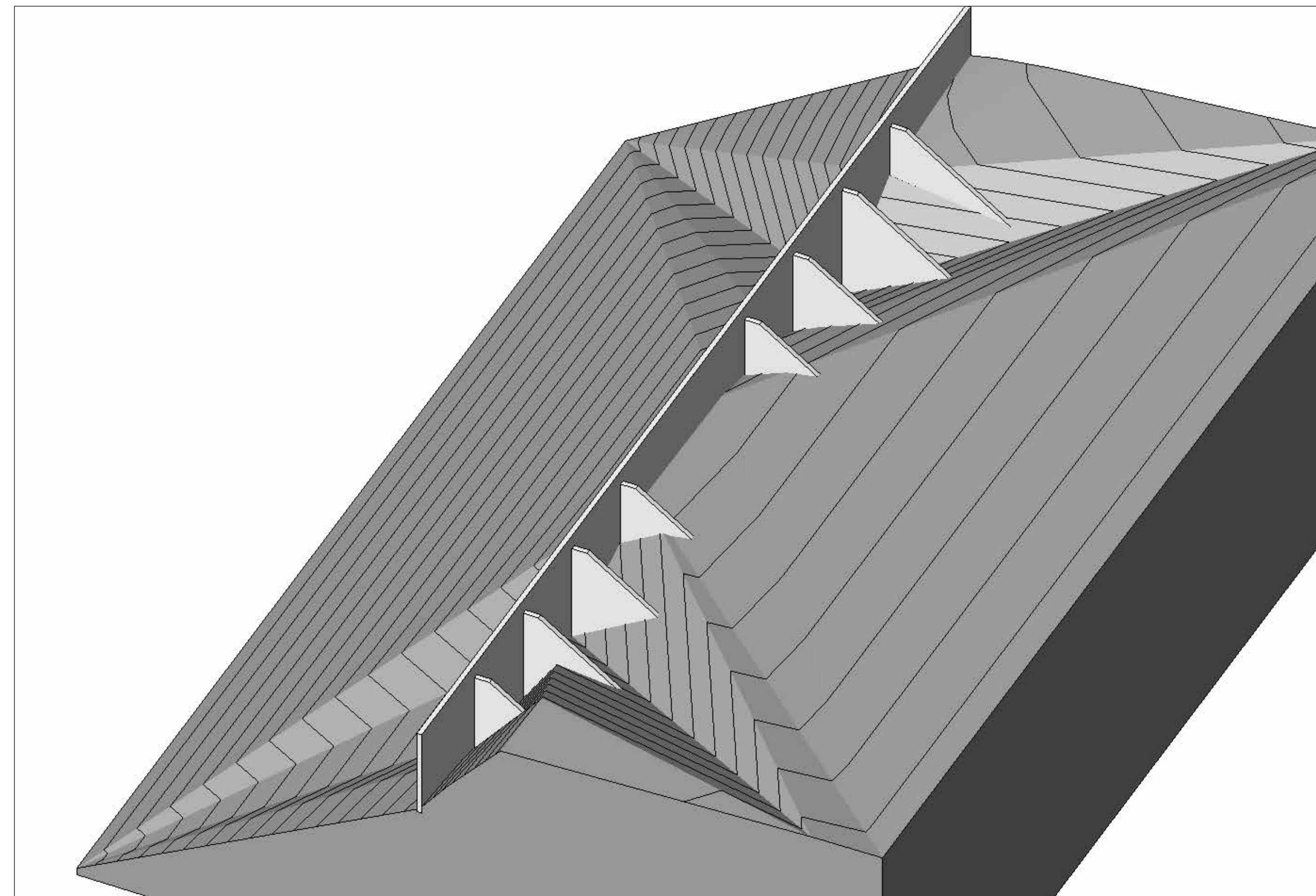
3D visning av prosjertert støttemur, med ribber forankret til fjell (figuren viser registrerte fjelldybder).
