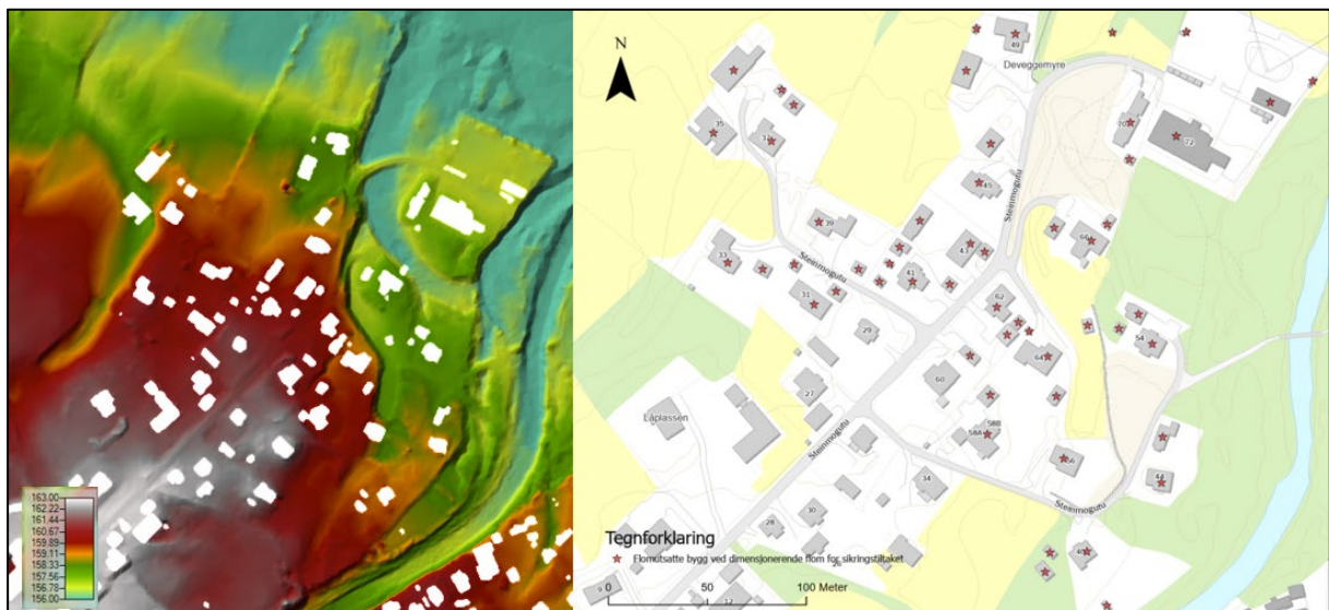
Figur 3. Terrengflata ved Steinmogutu til venstre og flomutsatte bygg ved dimensjonerende flom for sikringstiltaket.
