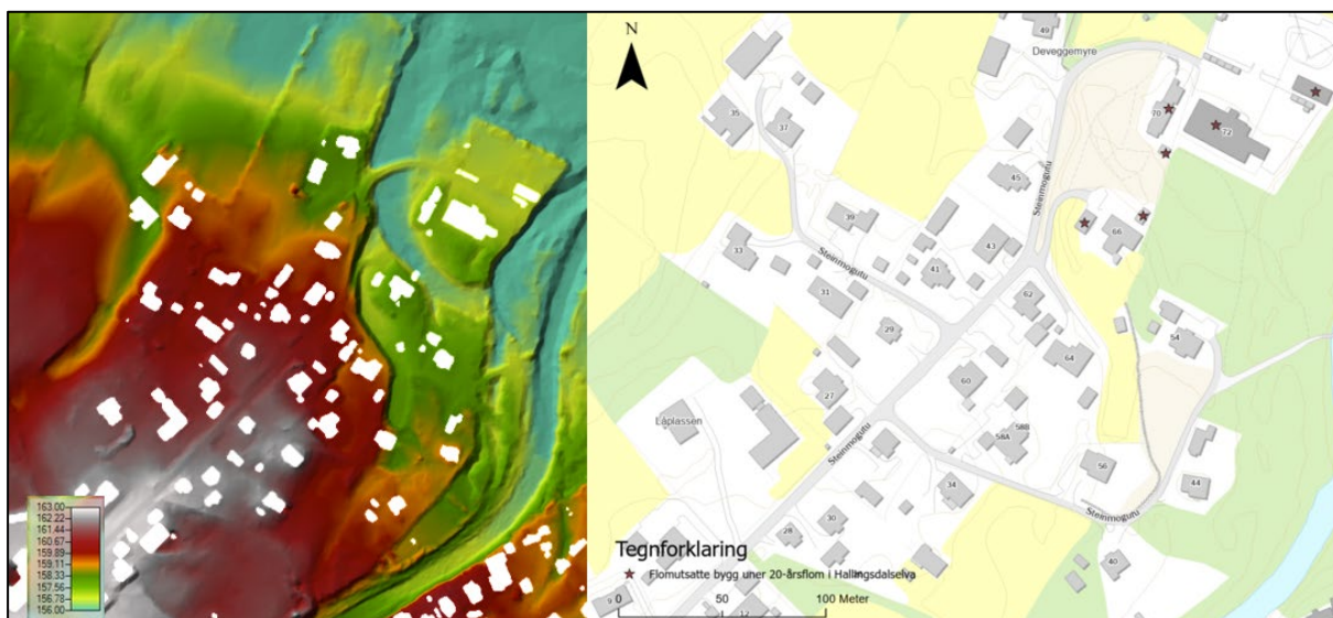
Figur 5. Terrengflata ved Steinmogutu til venstre og flomutsatte bygg ved 20-årsflom i Hallingdalselva
