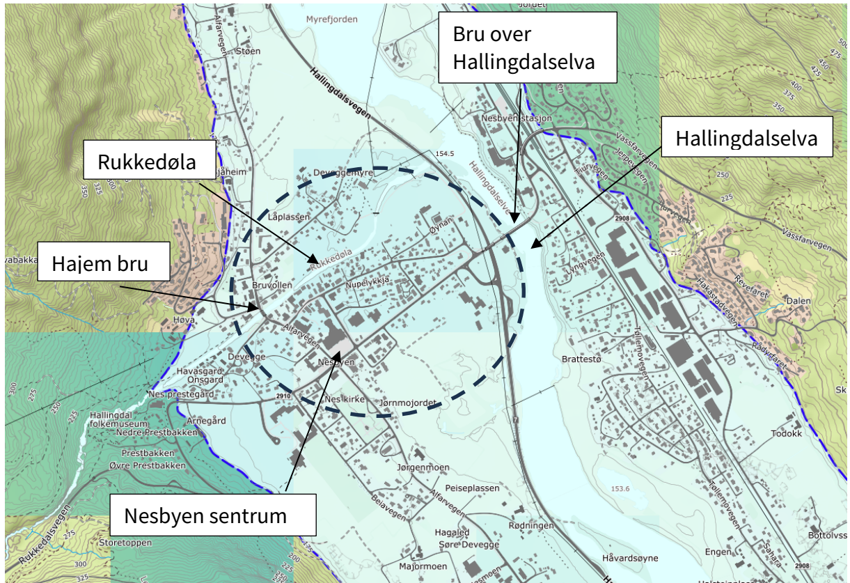
Figur 1: Oversikt over marin grense og mulighet for marin leire fra NGU. Planområdet grovt sett innenfor stiplede sirkel
