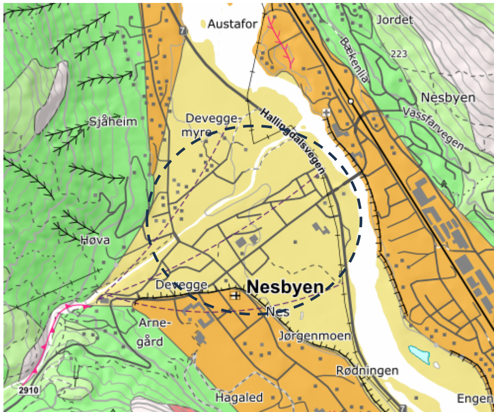
Figur 3: Løsmassekart fra NGU
