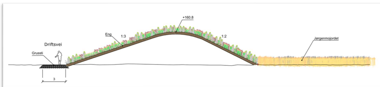
Figur 53. Prinsippsnitt for flomvullen over Jørgenmojordet uten turveg. Kilde: Rambøll
