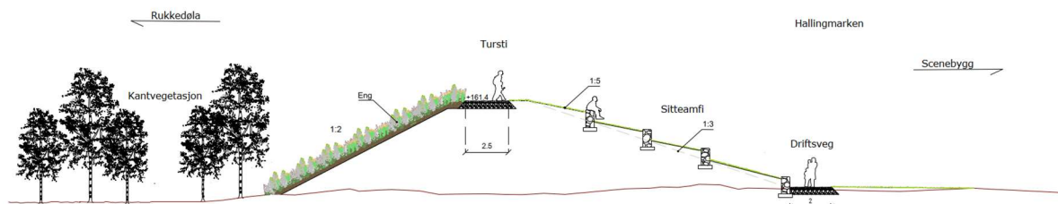
Figur 55. Prinsipsnitt for flomvoll langs Rukkedøla ved Hallingmarken. Bredde på driftsvei/turvei er ikke oppdatert. Kilde: Rambøll
