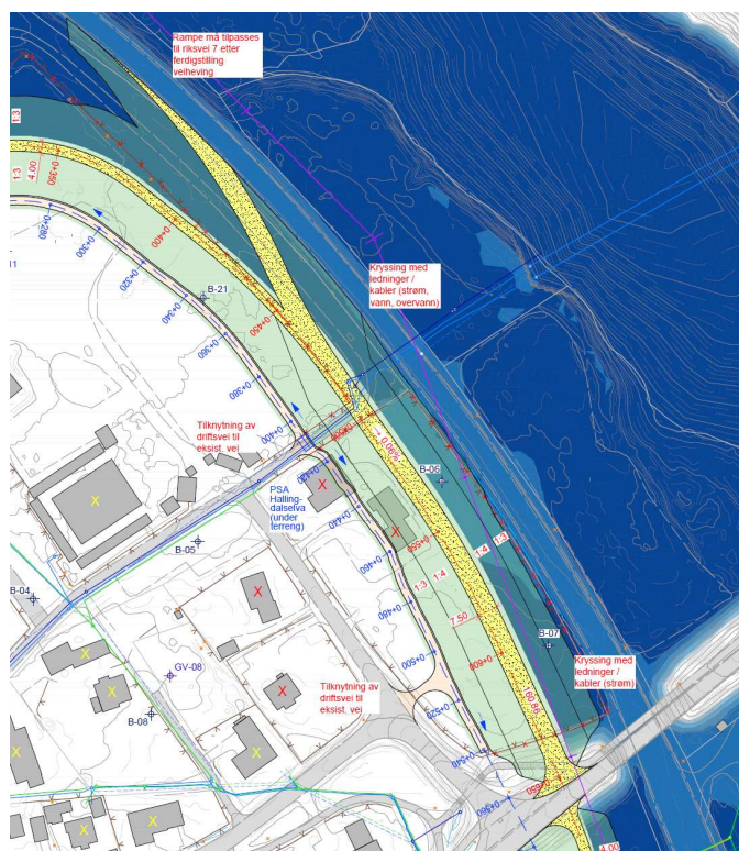
Figur 51. Strekning hvor flomvullen er planlagt kombinert med nødrampe til/fra Rv. 7, for bruk under flomhendelser. Utsnitt fra situasjonsplan, kilde: Dr. Blasy - Dr. Øverland Ingenieure GmbH. Tilkobling til Rv. 7 vil detaljeres senere av Statens Vegvesen.
