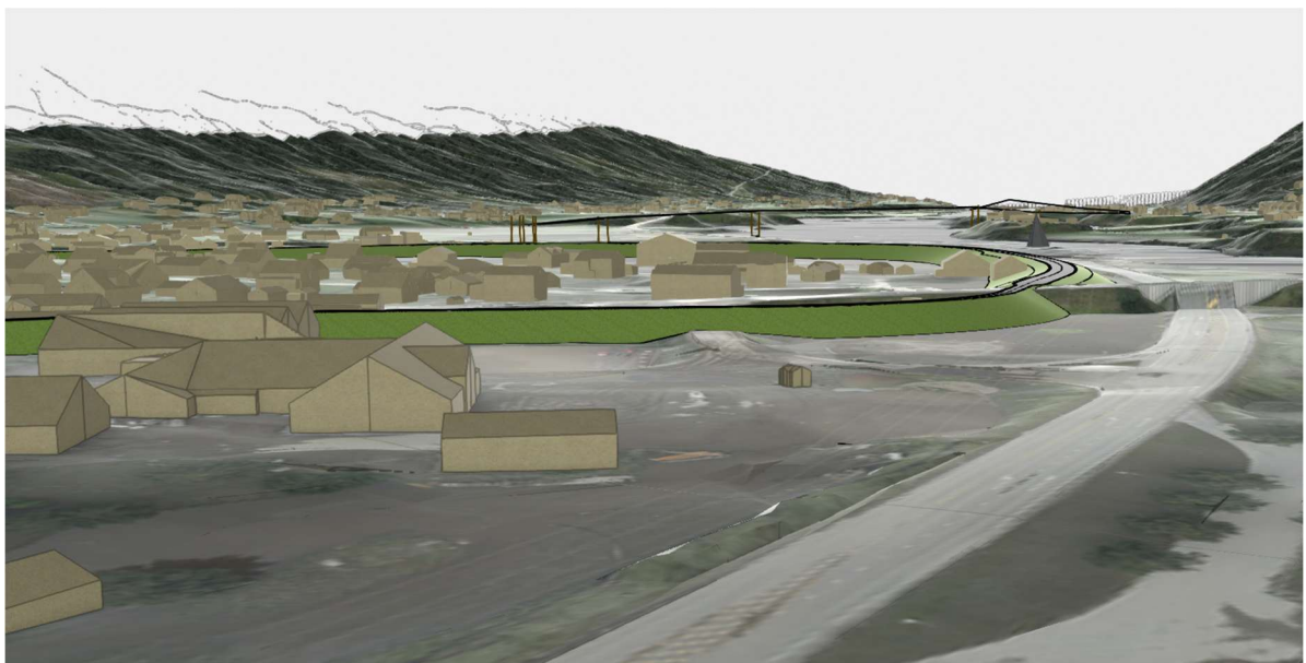
Figur 86. Utsnitt fra 3D-modell som viser flomvallen i mørkt grønt. Sett fra Rv. 7, mot nordvest.
