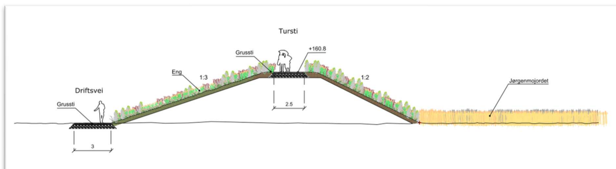
Figur 52. Prinsippsnitt for flomvullen over Jørgenmojordet med turveg. Bredde på driftsvei/turvei er ikke oppdatert. Kilde: Rambøll
