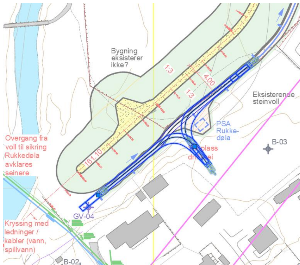
Figur 14 Sporingsberegning vendehammer.
