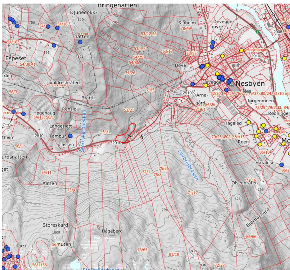
Figur 20. Kartutsnitt fra kartdatabasen (Granada). Blå sirkler viser registrerte grunnvannsborehull i fjell og gulesirkler er borehull i løs masser. Omtrentlig plassering av masseuttaket er vist med omriss.
