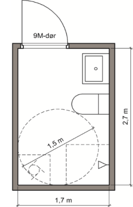
Fig. 6 c Baderom med litt bedre plassforhold og utstyrsplassering enn rommet i fig. 6 b
