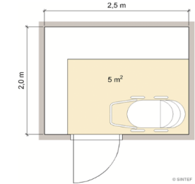
Fig. 54 Eksempel på sportsbod på 5,0 m² Døra er plassert på langsiden av boden og er trukket ut fra sideveggen.
