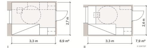
Fig. 53 I Rom med enkeltsg. Med en rombredde på 2,7 m blir det mulig å møblere langs begge langveggene, noe som gjør rommet mer funksjonelt. II Rom med enkeltsg. Hvis arbeidsbordet sløyfes, blir det fri passasje på 0,9 m fram til vinduet. Døra er plassert 0,35 m ut fra veggen, slik at det er mulig å sette en bokhylle bak døra.
