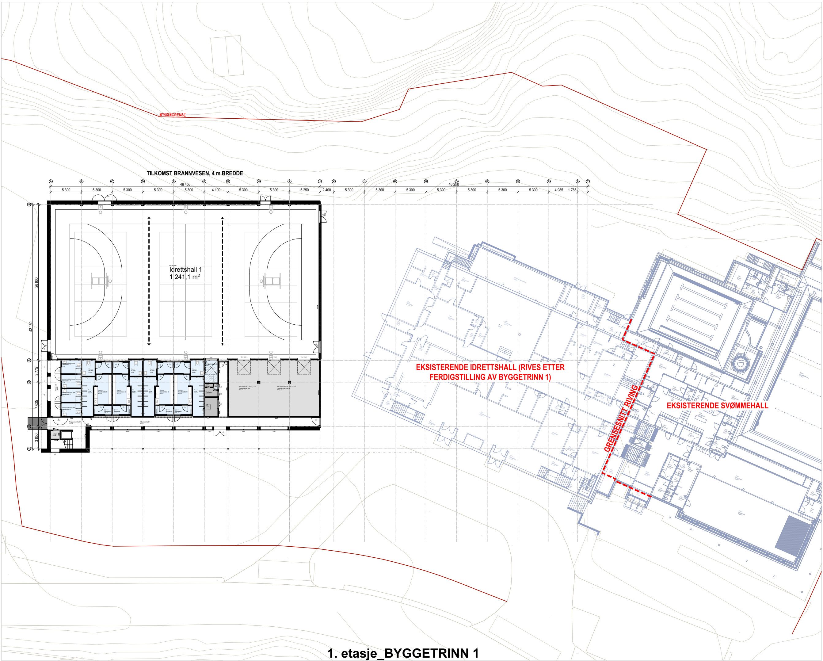
1. etasje_BYGGETRINN 1
