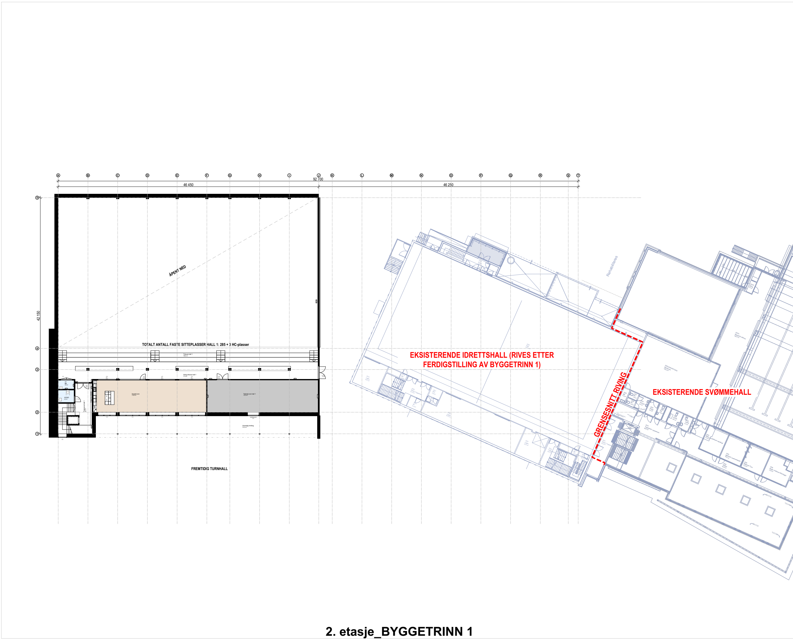
2. etasje_BYGGETRINN 1
