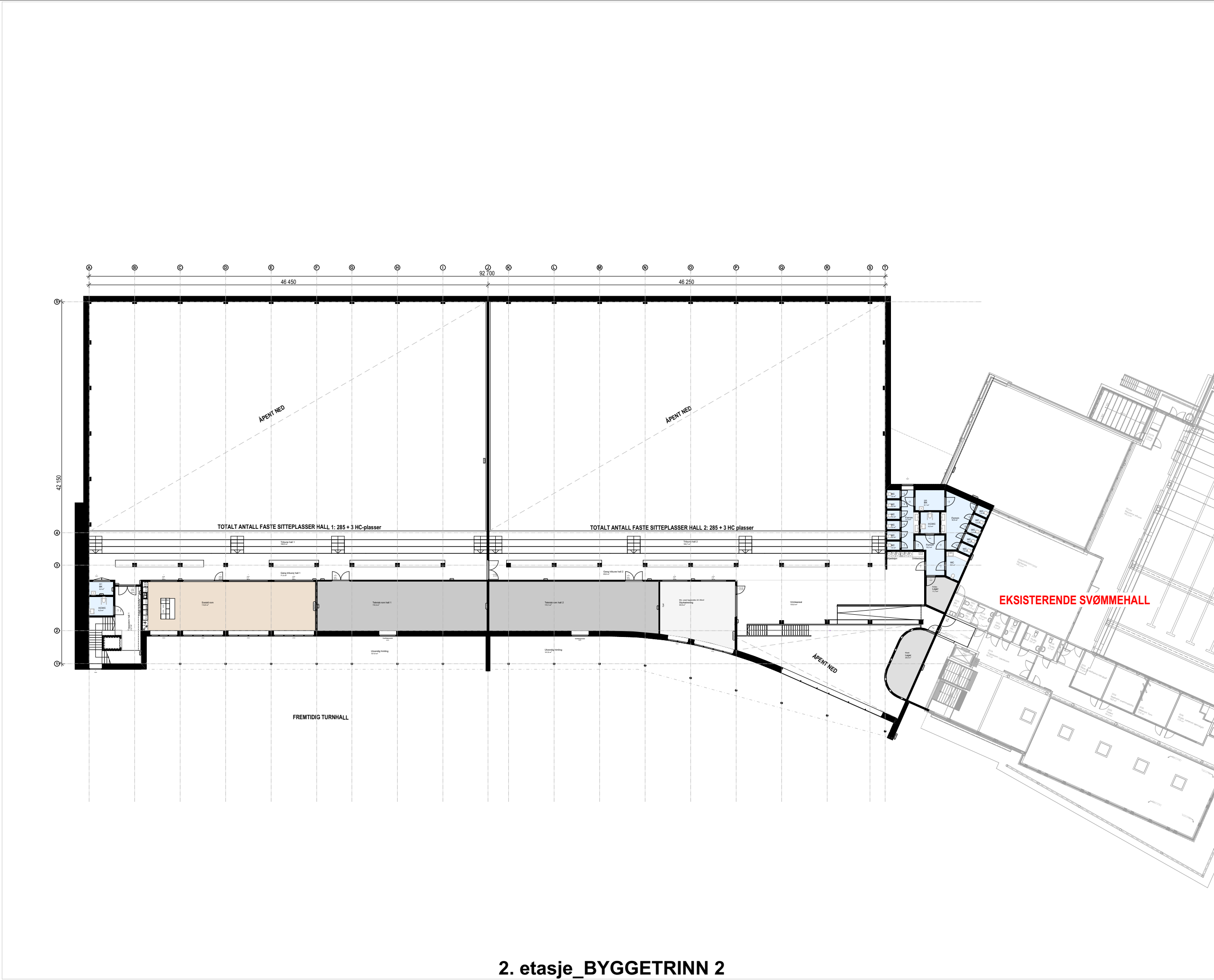
2. etasje_BYGGETRINN 2
