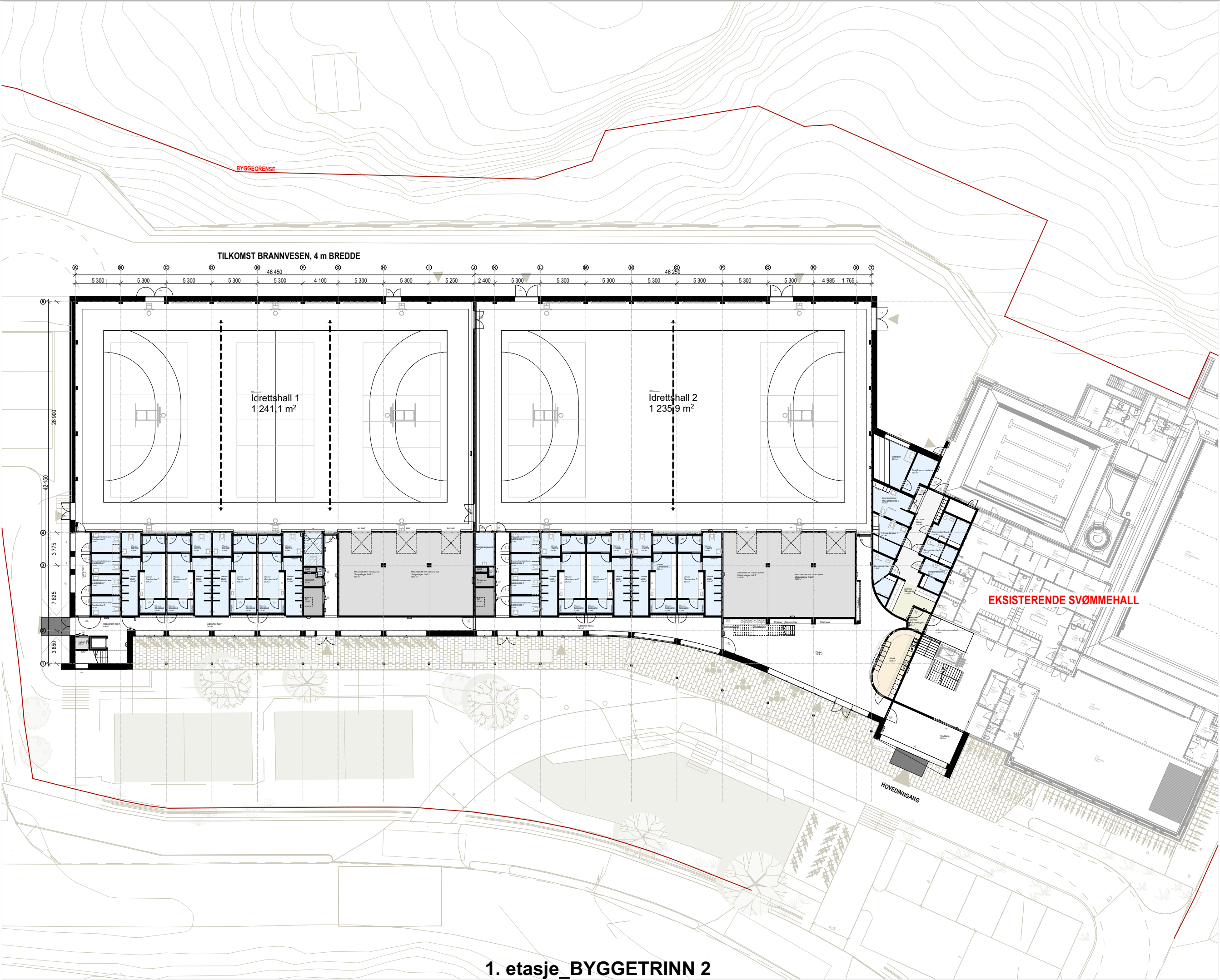
1. etasje_BYGGETRINN 2
